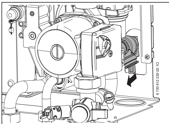
Bild 92 Sicherheitsventil (Heizung)
