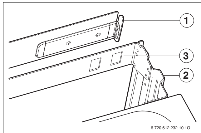
Bild 11 Einhängen des Geräts an der Aufhängeschiene
