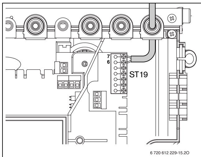
Bild 18 Anschluss Regler
