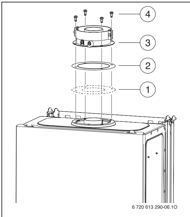
Bild 13 Drosselscheibe montieren
