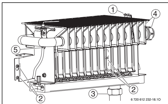
Bild 83 Baugruppe Brenner
