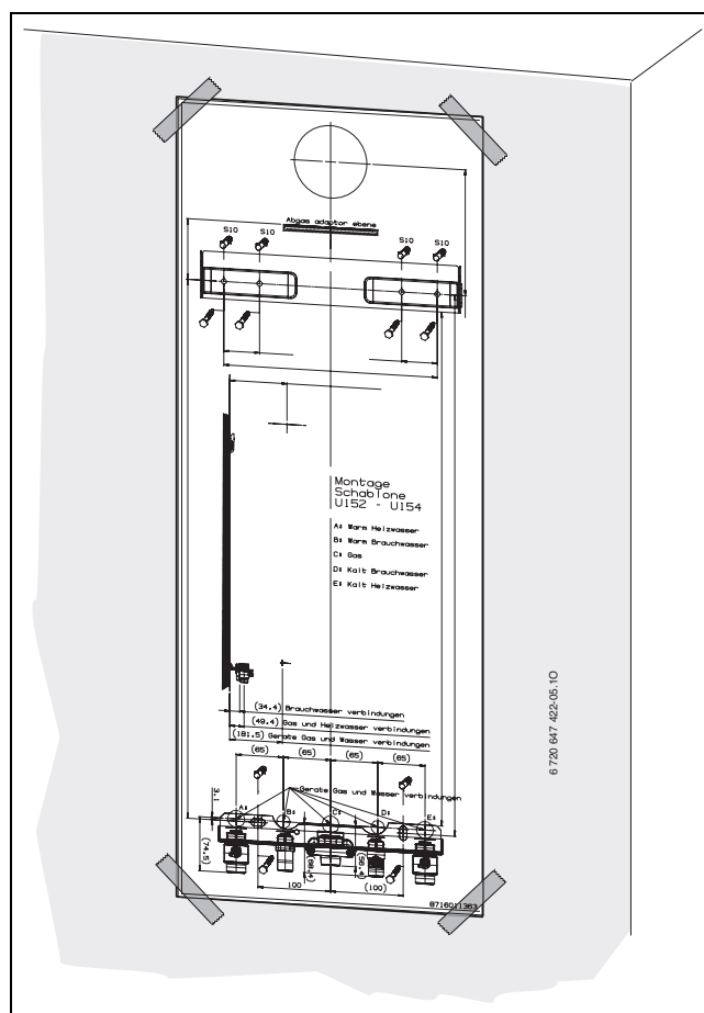
Bild 8 Montageschablone
