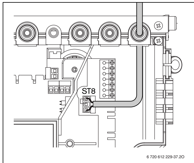
Bild 22 Anschluss Speicherthermostat
