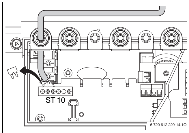
Bild 17 Anschluss Easyswitch
