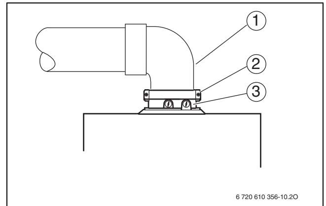
Bild 14 Befestigung des Abgaszubehörs mittels Schelle
